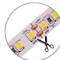
Corte 50mm
